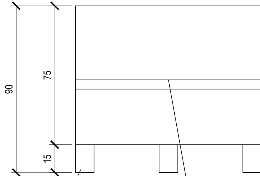
VISTA INTERNA
