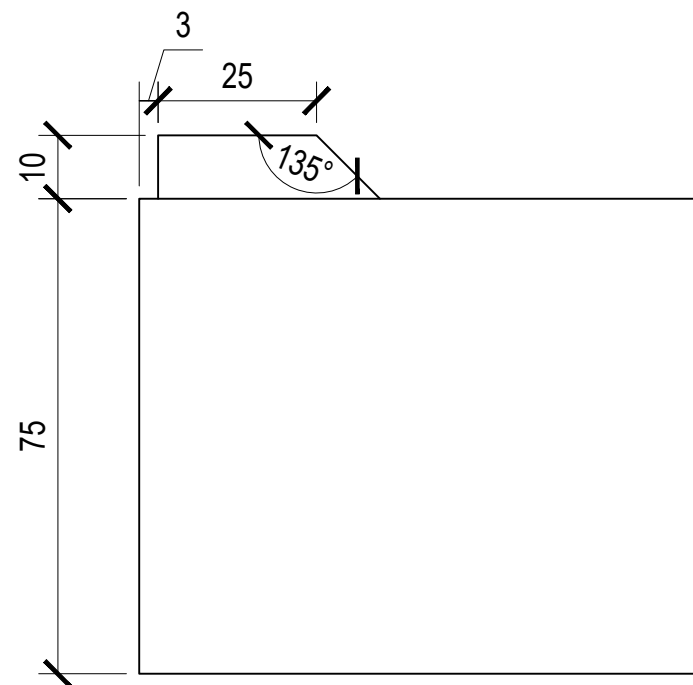
VISTA LATERAL ESQUERDA MESA PLENÁRIO ESC - 1:20
