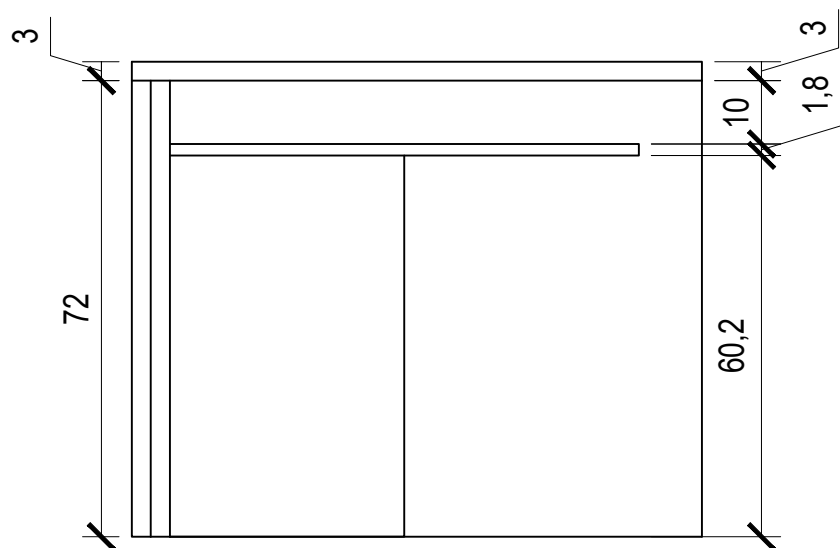
CORTE ESC - 1:20
