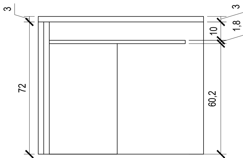
CORTE ESC - 1:20
