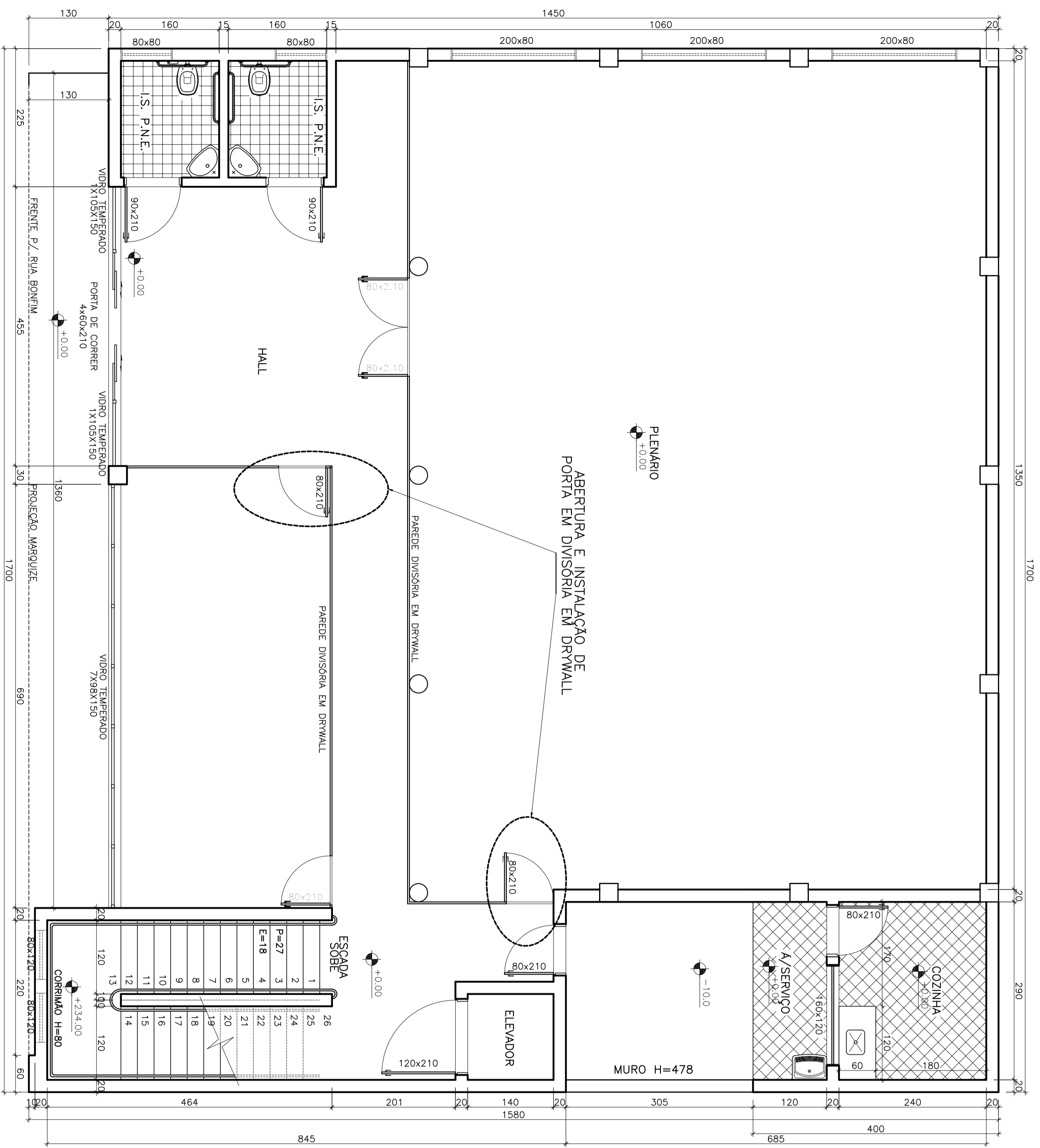
PLANTA BAIXA TIPO PAVIMENTO TÉRREO ESCALA 1 / 50
