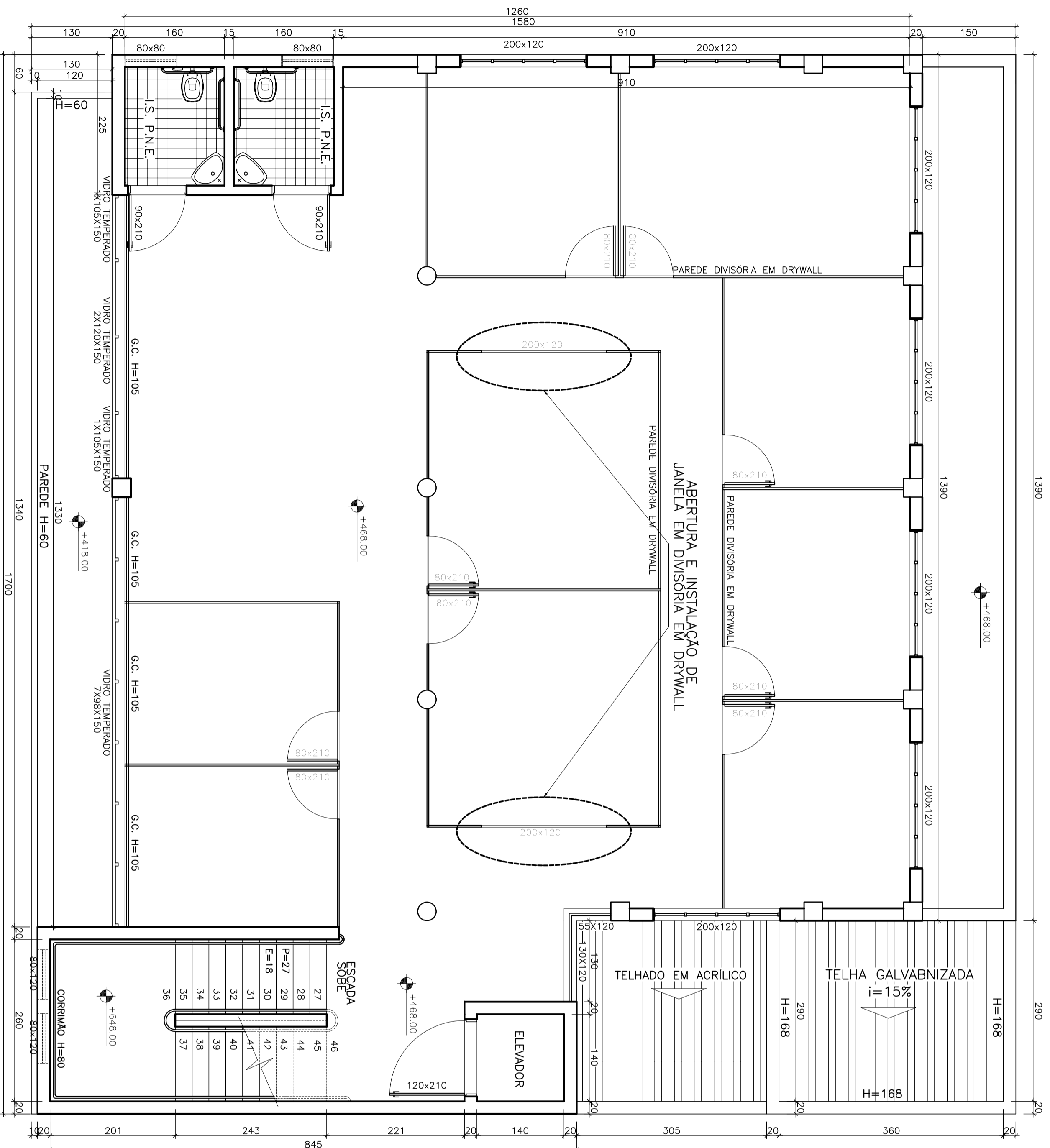
PLANTA BAIXA TIPO 2º PAVIMENTO ESCALA 1 / 50
